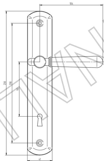
DASA NOVA KLIKA DOZ 90mm PRAVA-MS-BR
