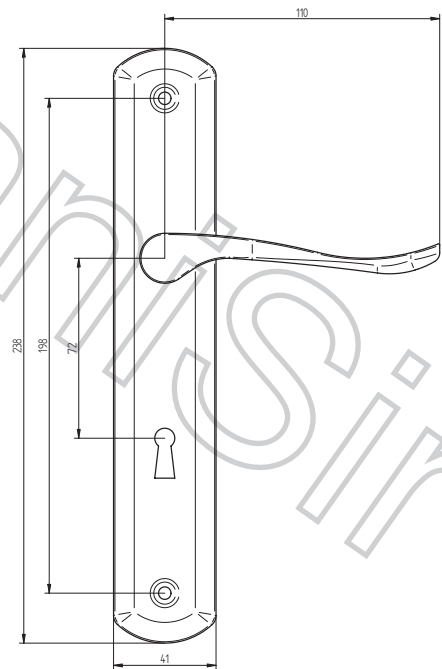
ELA NOVA KLIKA DOZ 72mm PRAVA-MS-BR
